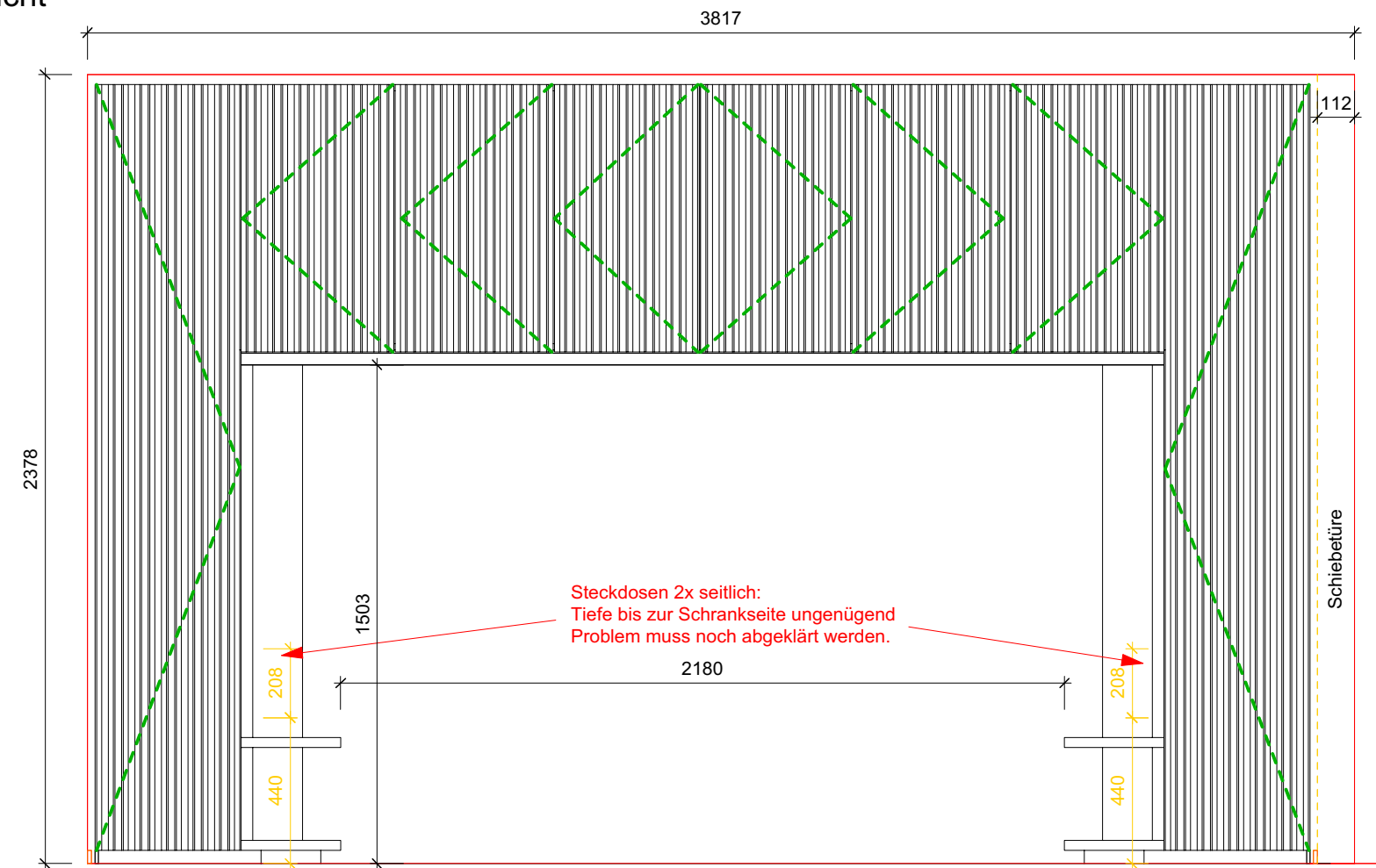
Ansicht
