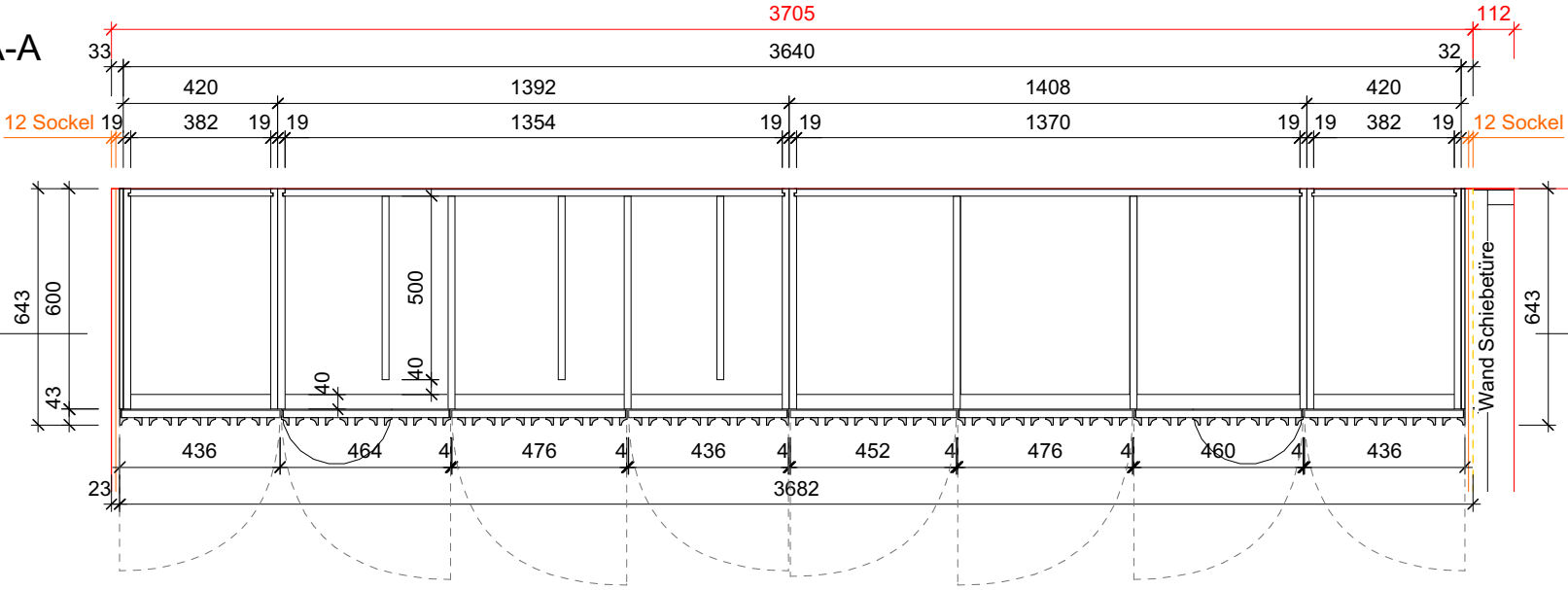
Ansicht
